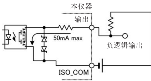
负逻辑输出
