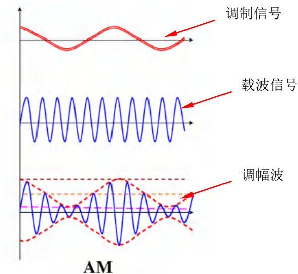
图 17-10 调幅
