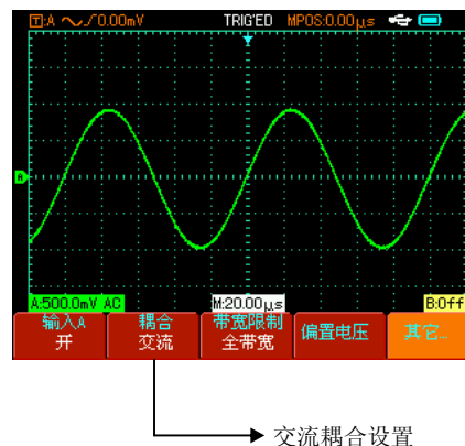
图2-7 只显示被测的交流信号
