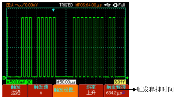
图2-16 触发释抑
