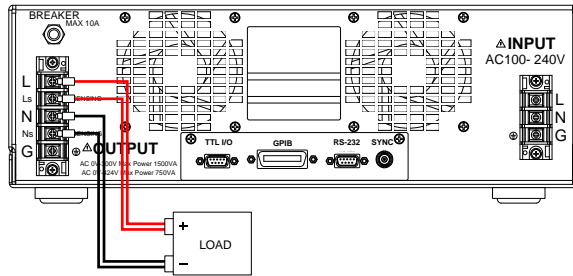
输出连接示意图
