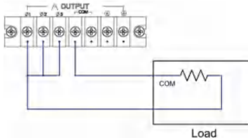
单相输出连接示 意图
