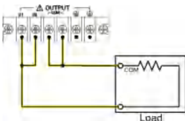
并联输出连接示意图
