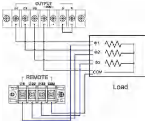
三相输出与遥测 连接示意图
