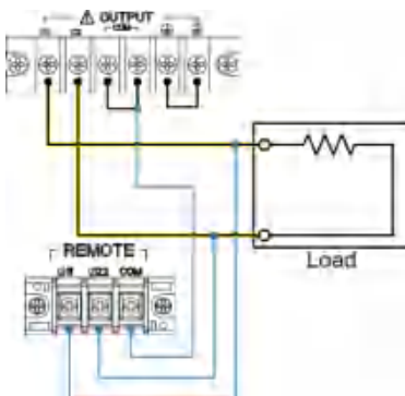
输出与遥测连接示意图
