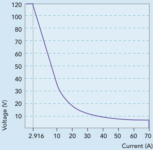
型号 63123A 输入特性
