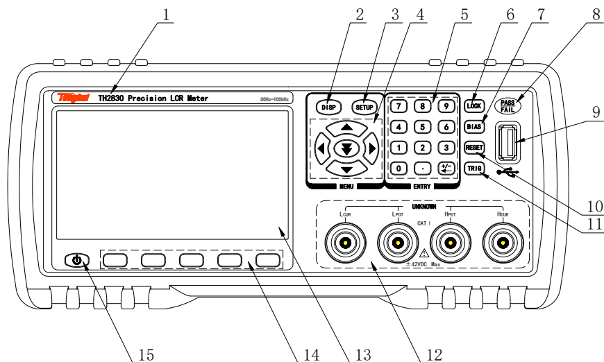
图 2-1. 前面板说明
