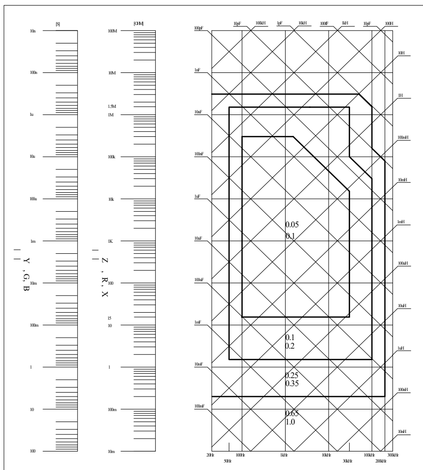
图 A 基本测量准确度 A
