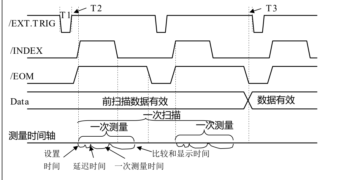
图 8-5 计时图解
