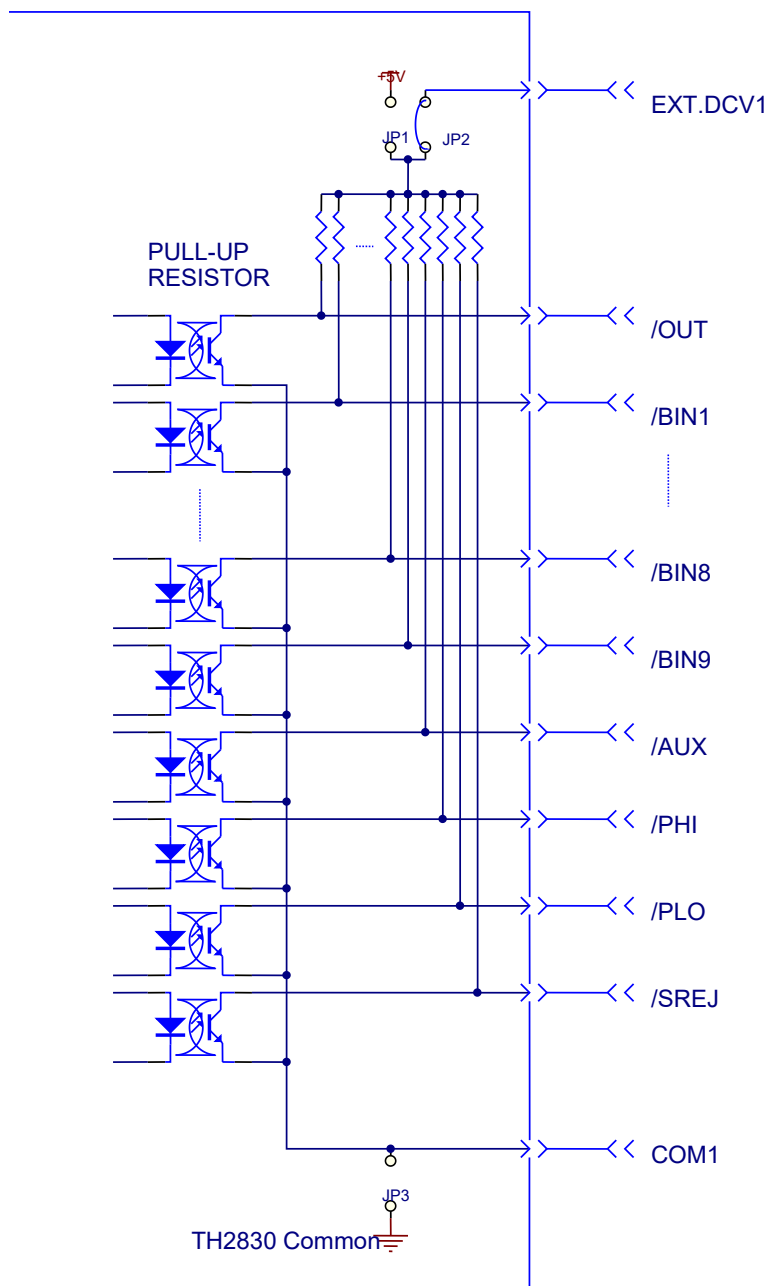
比较结果信号输出电路
