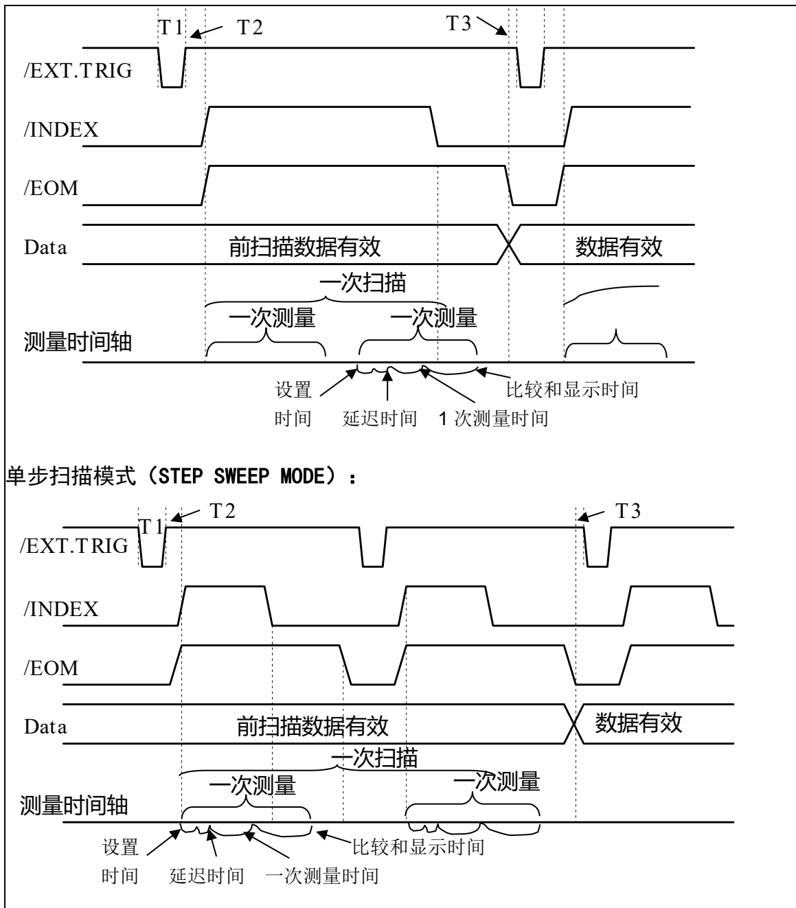
图 8-5 计时图解
