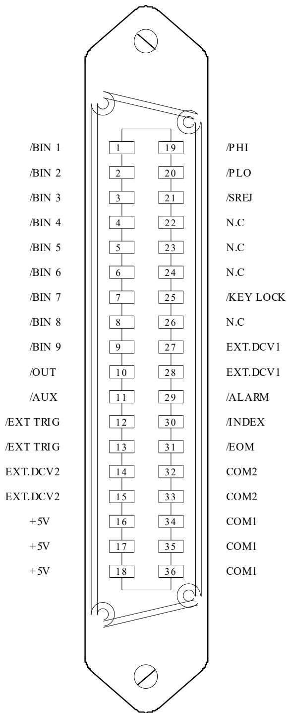
图 8-2 HANDLER 连接接口管脚定义
