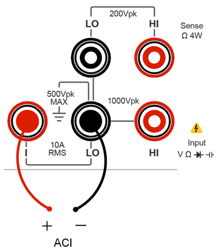
图 5.13 交流电流测量连接示意图
