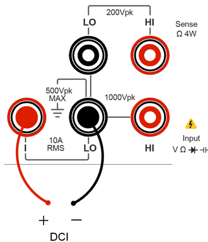
图 5.7 直流电流测量连接示意图
