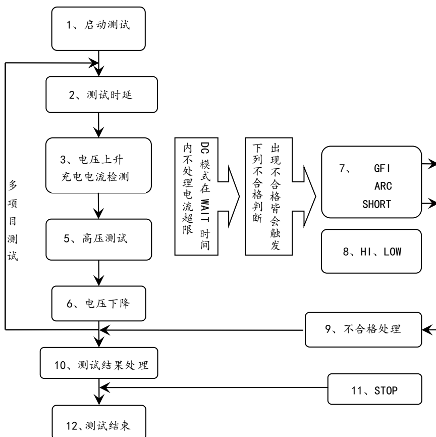
仪器的测试流程框图
