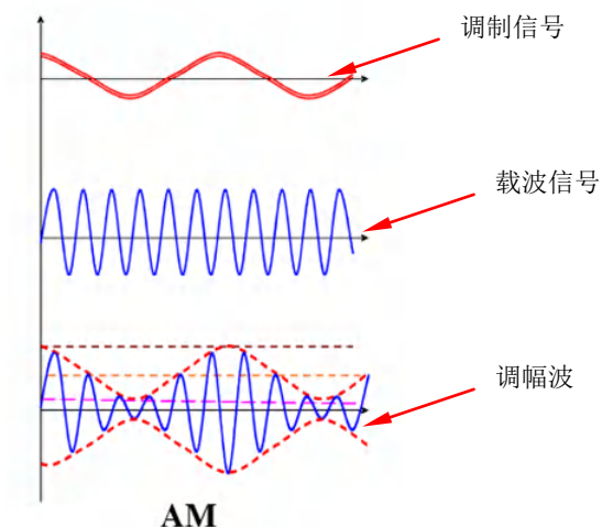
图 13-9 调幅
