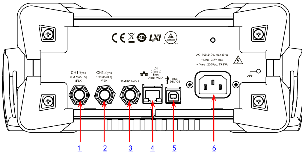
图 1-2 后面板
