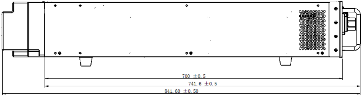
IT7842E-350-210 机型
