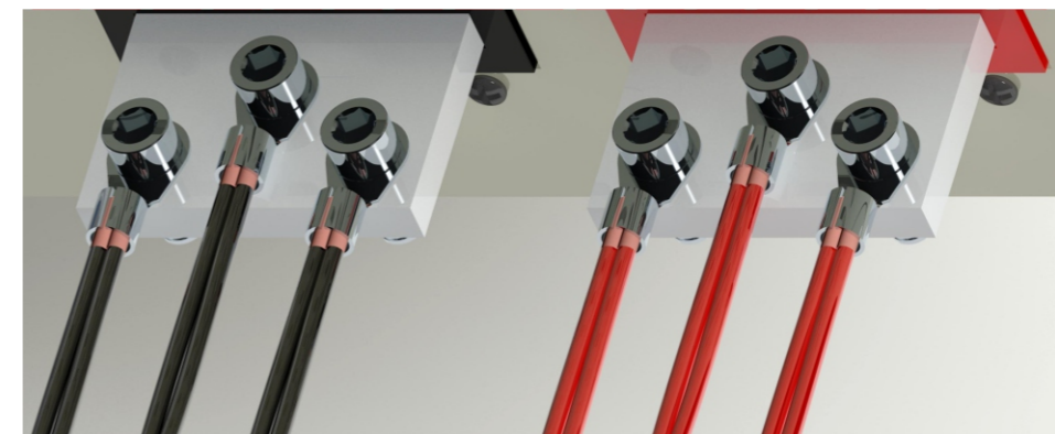
图 4-3 使用接线铜排时的接线方式
