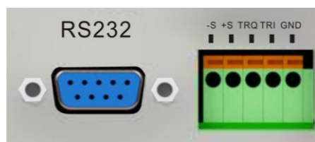
图 4-8 RS232 通信插座和多功能输入输出接线柱
