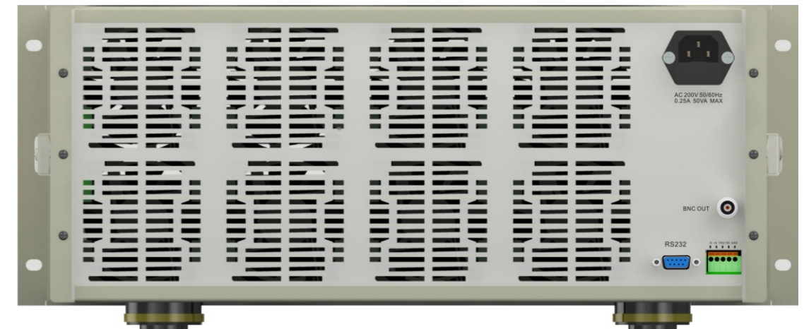
图 4-6 RK9715、RK9715B、RK9716 和 RK9716B 后面板
