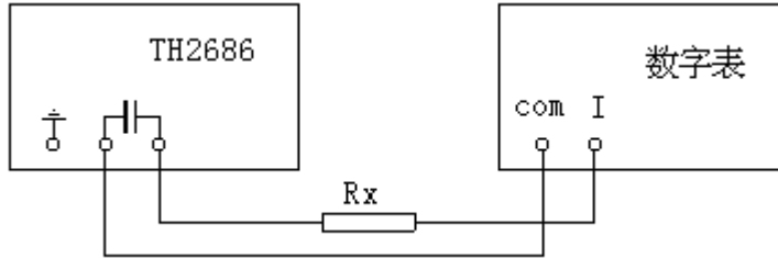
图 5 漏电流的校准与检验
