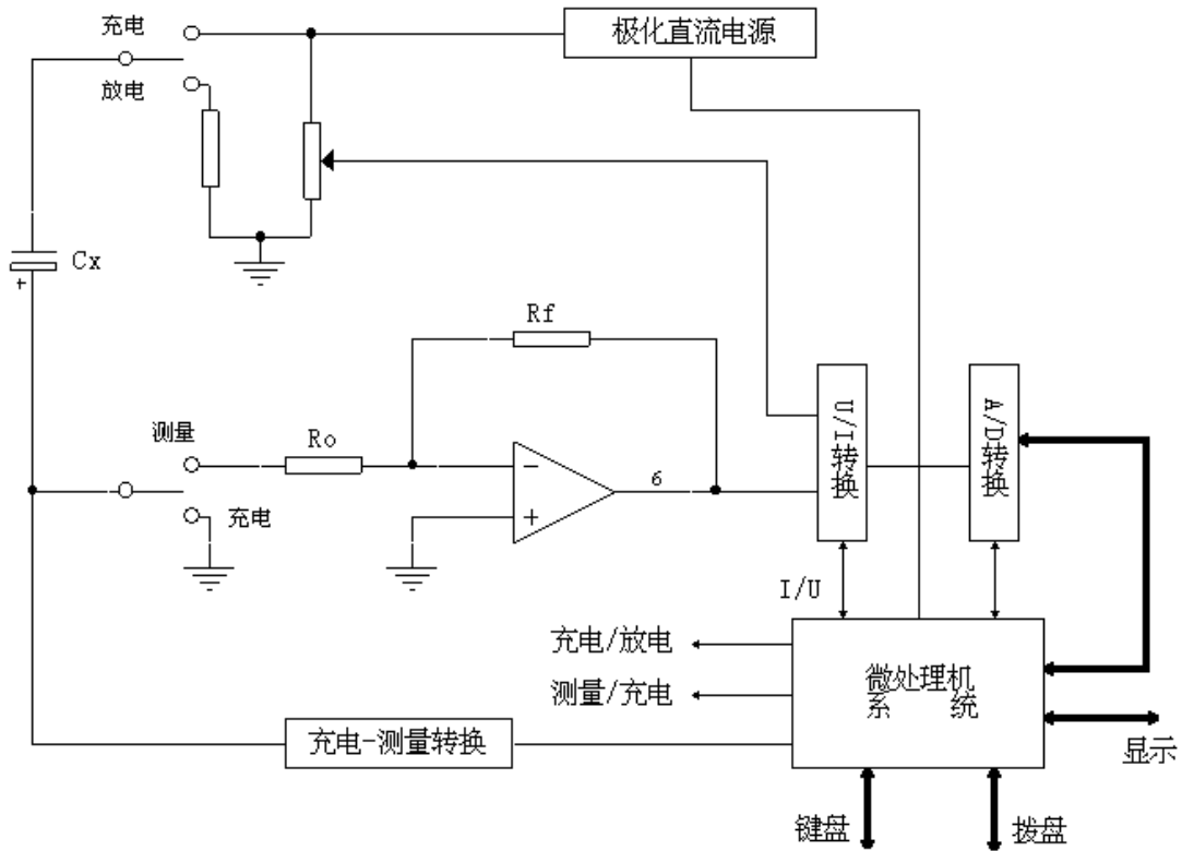
图 2 仪器框图
