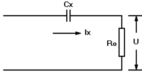
图 1 测量原理
