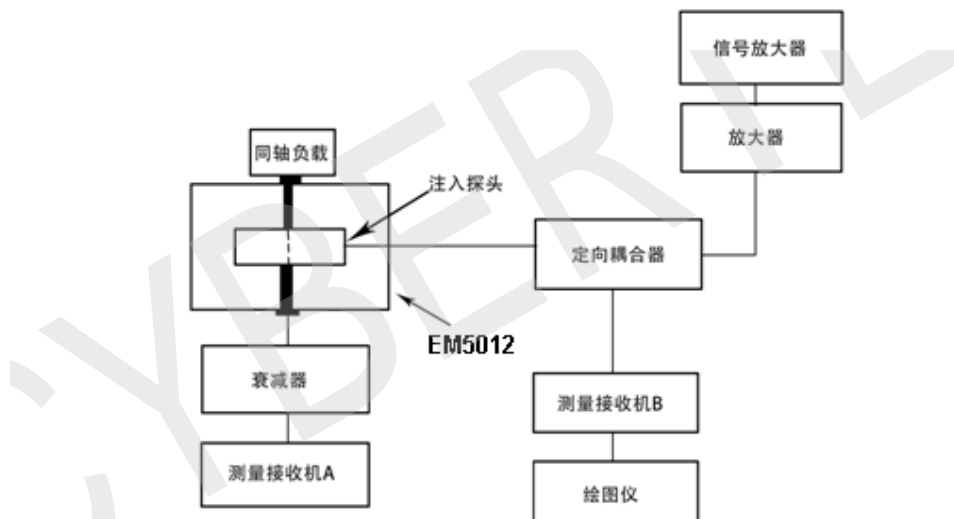
◇ GJB152A-97 中 CS115 电流探头校准图
