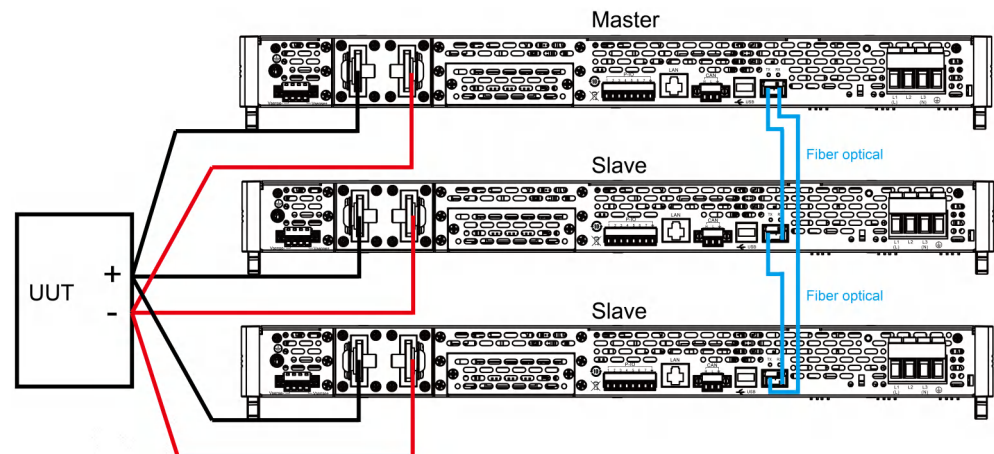
图 5-1 线路连接图
