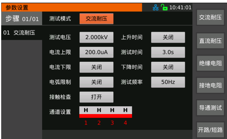
图 3-13-4 通道配置
