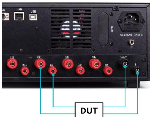
图 3-20-1 接地通道连线
