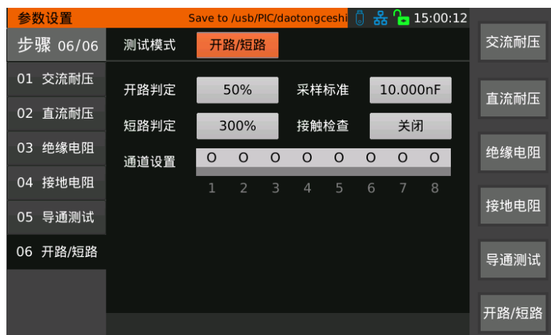
图 3-23 开路短路测试设置
