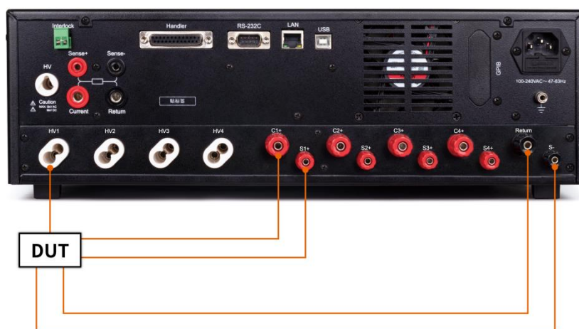
图 3-18-3 同步测试连线
