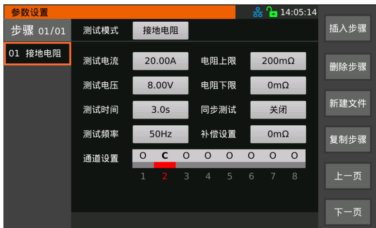
图 3-21 接地通道设置
