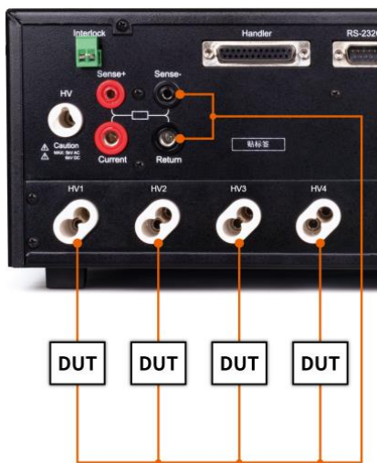
图 3-13-5 测试接线
