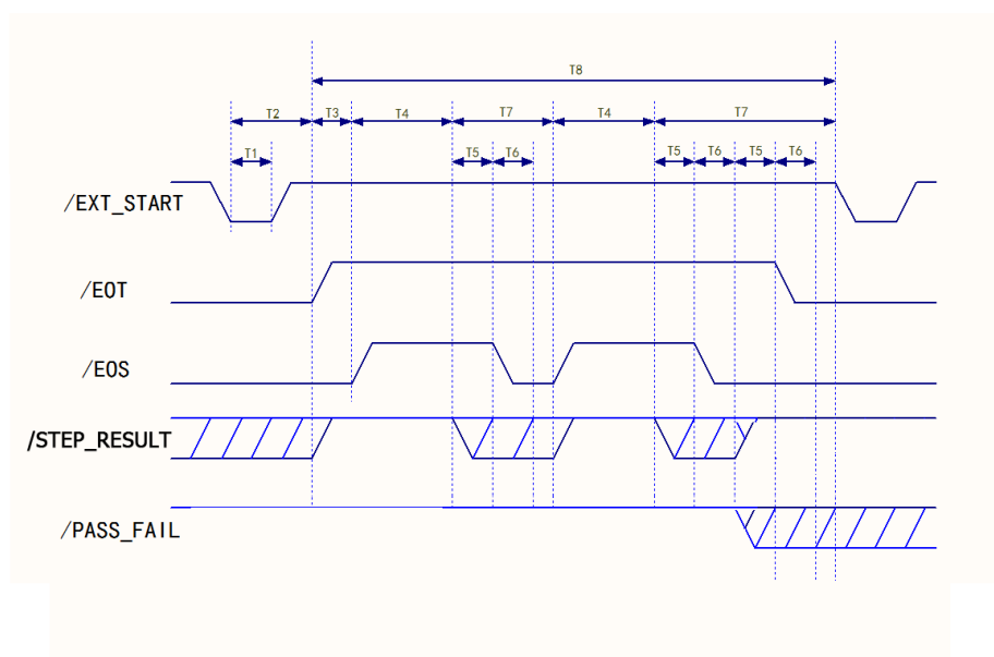
时序图——以 2 个测试步骤为例
