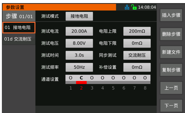
图 3-19 接地电阻同步测试通道设置
