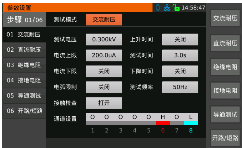
图 3-13 交流耐压参数设置
