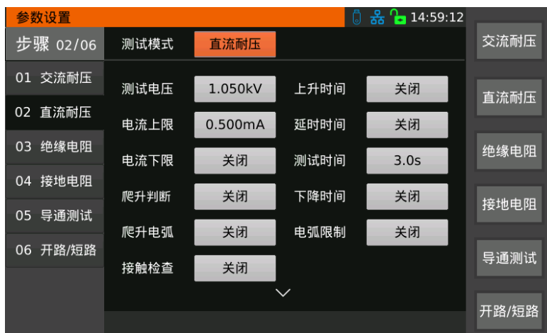
图 3-14 直流耐压设置 1
