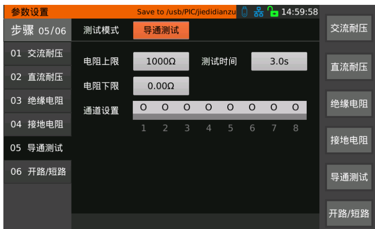
图 3-22 导通测试设置
