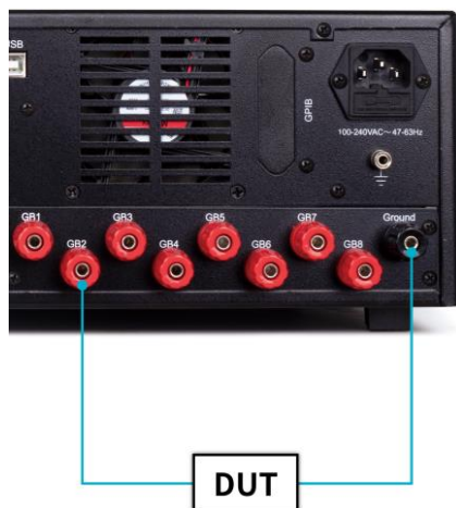
图 3-21-1 接地通道连线
