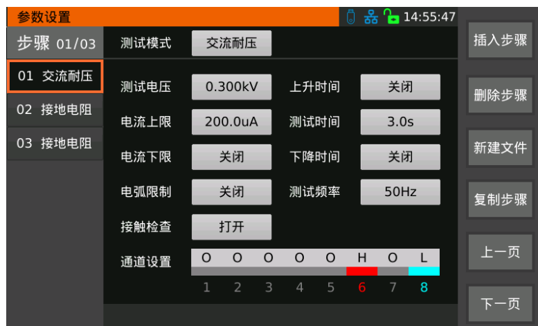
图 3-11 测量设置
