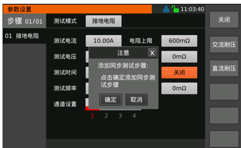
图 3-18-1 接地电阻与交流耐压同步测试
