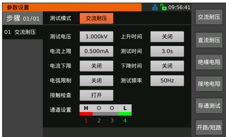
图 3-13-1 通道配置
