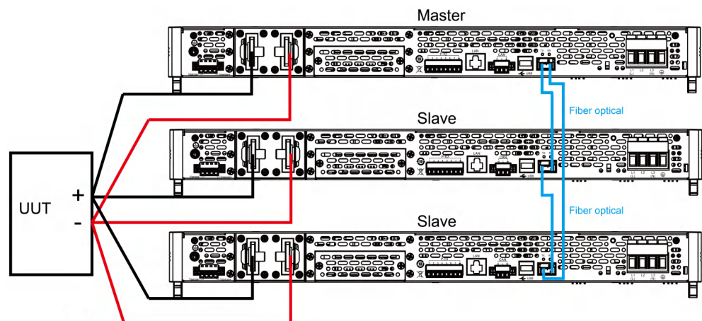
图 5-1 线路连接图
