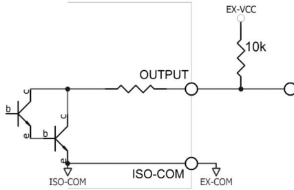
图9-2-6-3负逻辑输出
