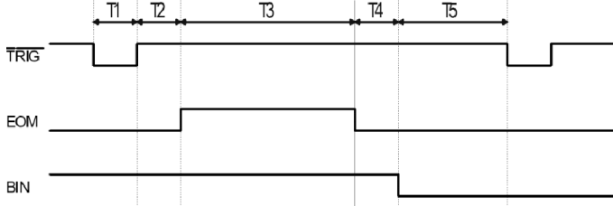
图9-3-1周期表
