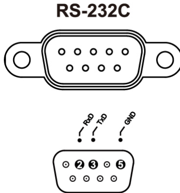
图 10-1-1后面板上RS-232接口[公头]
