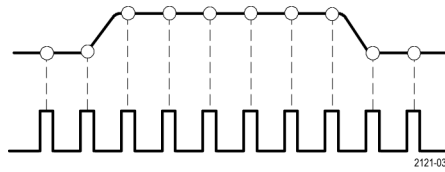
取样速率
