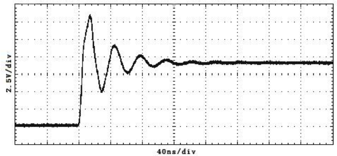
添加输入延长线(CK-301)的波形
