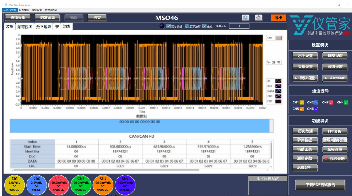
图 5.1 - 1 功能（二十二）CAN总线解码
