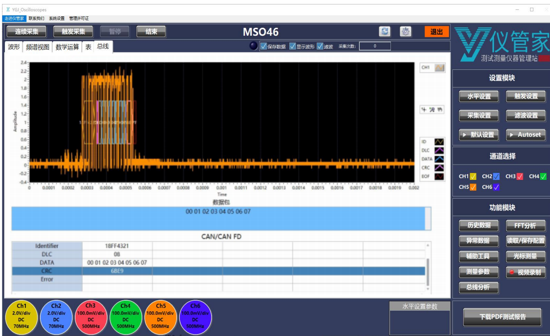
图 5.1 - 2 功能（二十三）CAN-FD总线解码
