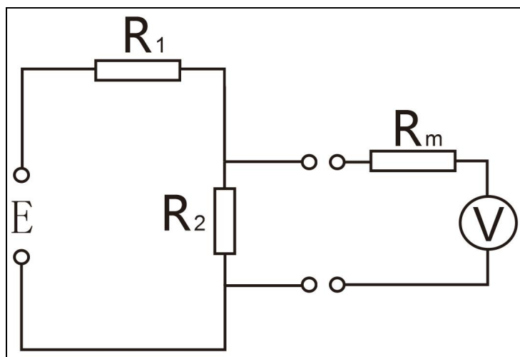
图 5-32 负载效应
