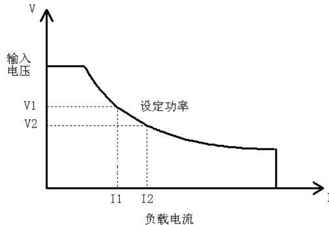
图 5-10 恒功率模式
