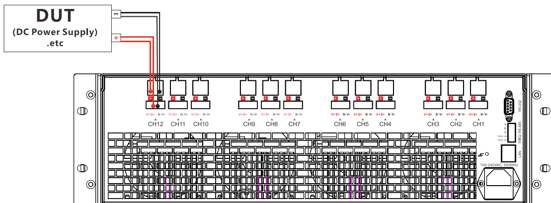
图 3-3 远端采样连接
