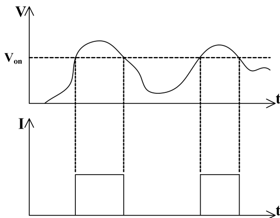
图 5-45 非锁定 V_{on} 带载
