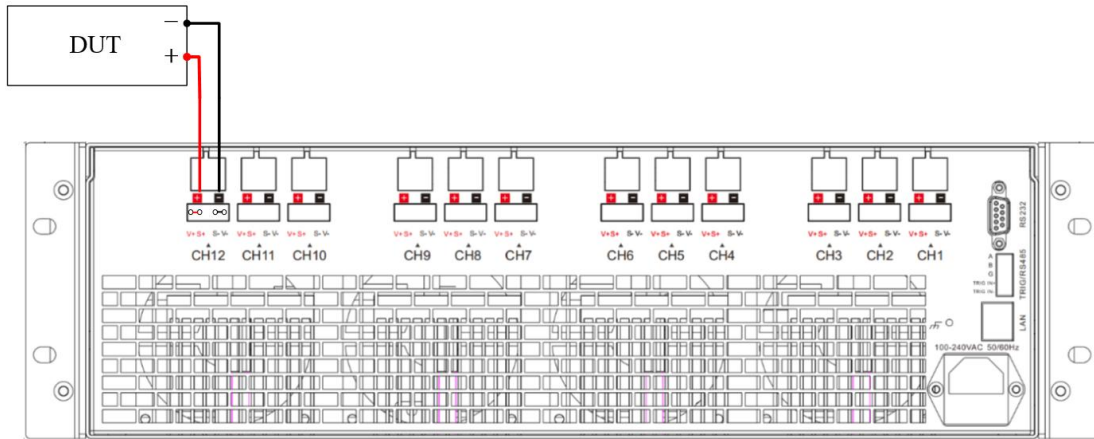
图 3-1 近端采样连接
