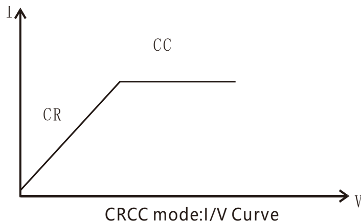
图 5-14 恒阻恒流模式
