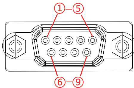
图 4-12 RS232 引脚标识
