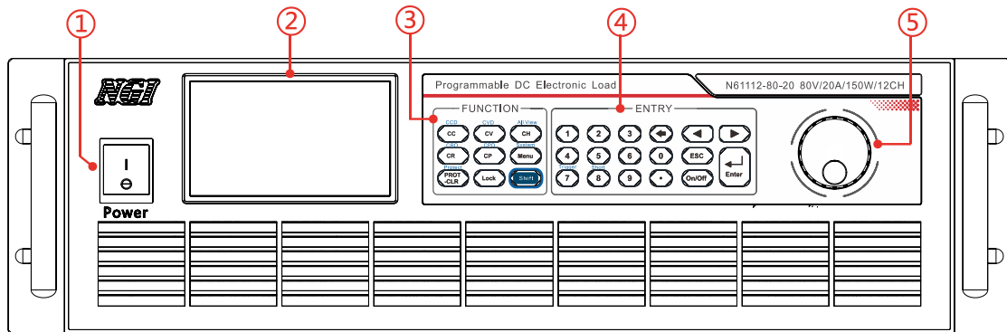
图 4-4 前面板
