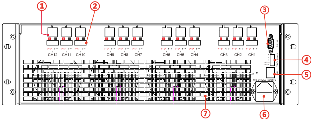
图 4-9 主机后面板—12CH
