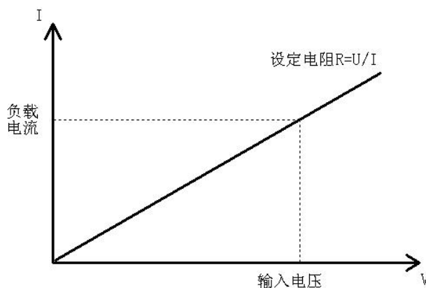
图 5-8 恒电阻模式
