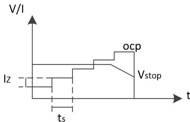
图 5-24 过流测试
