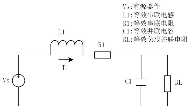
图 5-34 阻抗模拟
