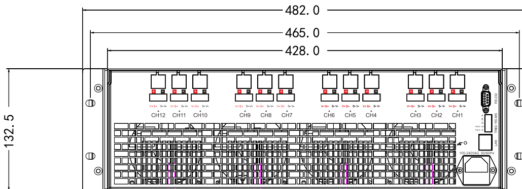
图 4-3 主机后面板尺寸—12CH (mm)
