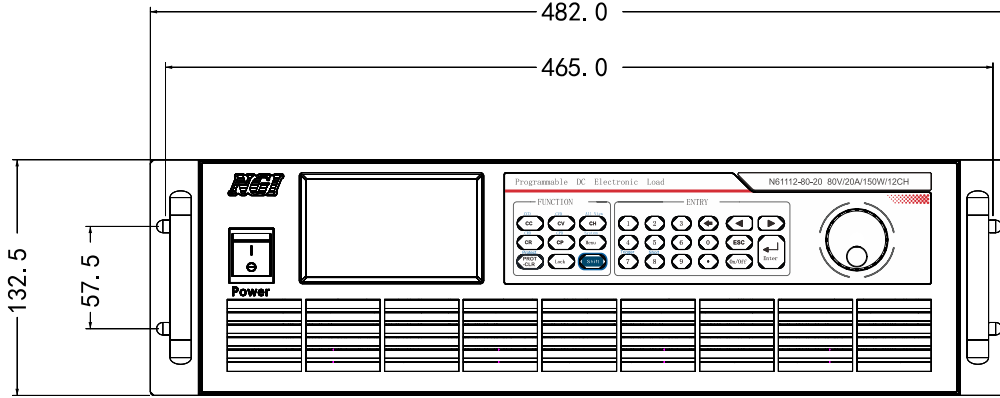
图 4-1 主机前面板尺寸 (mm)
