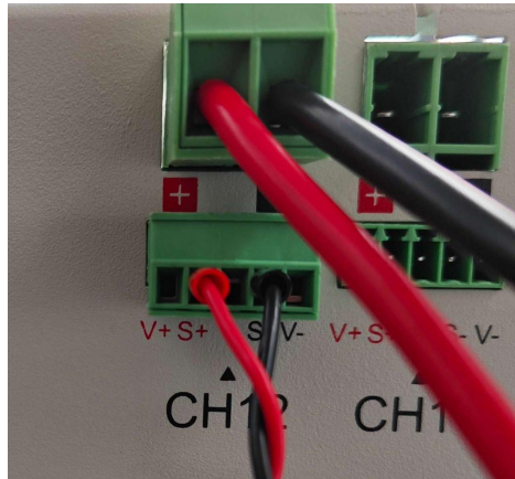
图 3-4 局部示意图
