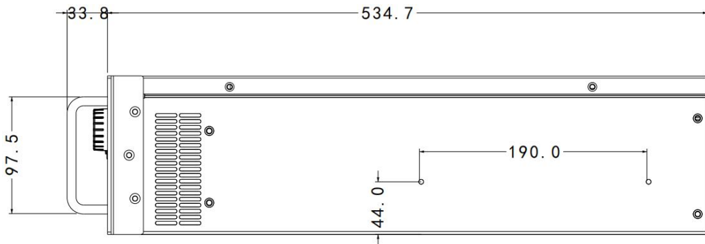
图 4-2 主机机箱侧视尺寸 (mm)
