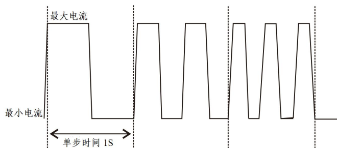
图 5-20 动态扫描
