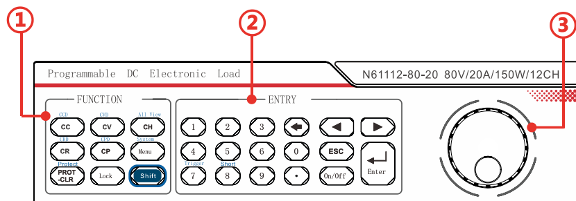
图 4-5 键盘
