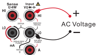
图 2-20 信号频率测量连接示意图
