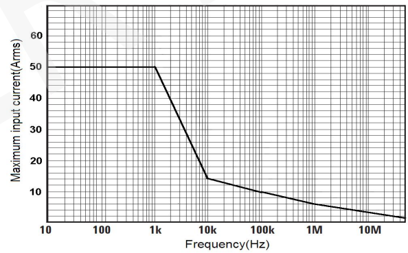
图 5 HCP8050 最大测量电流 VS 频率曲线 (超过该曲线所示最大电流连续使用会导致探头烧毁)
