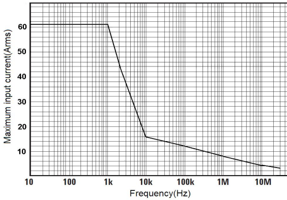
图 8 HCP8070 最大测量电流 VS 频率曲线 (超过该曲线所示最大电流连续使用会导致探头烧毁)
