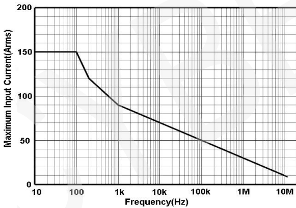
图 11.a HCP8150 最大测量电流 VS 频率曲线 (超过该曲线所示最大电流连续使用会导致探头烧毁)
