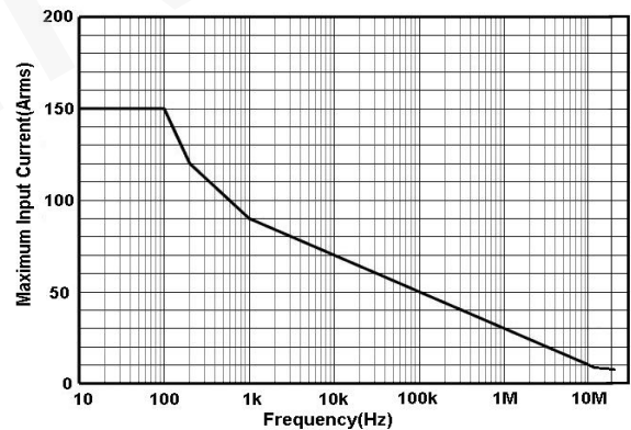
图 11.b HCP8150A 最大测量电流 VS 频率曲线 (超过该曲线所示最大电流连续使用会导致探头烧毁)
