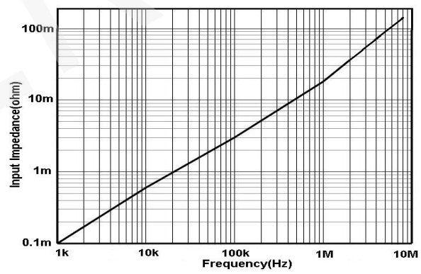
图 15.b HCP8300A 输入阻抗 VS 频率曲线
