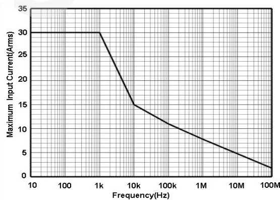
图 2.c HCP8030D 最大测量电流 VS 频率曲线
