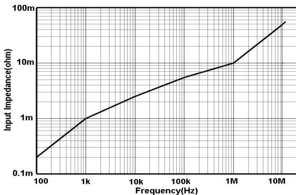
图 12.a HCP8150 输入阻抗 VS 频率曲线
