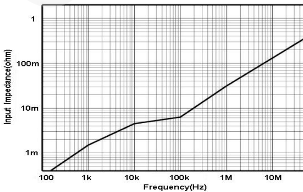
图 6 HCP8050 输入阻抗 VS 频率曲线
