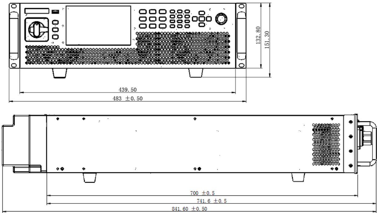
IT7942EP-350-210 机型
