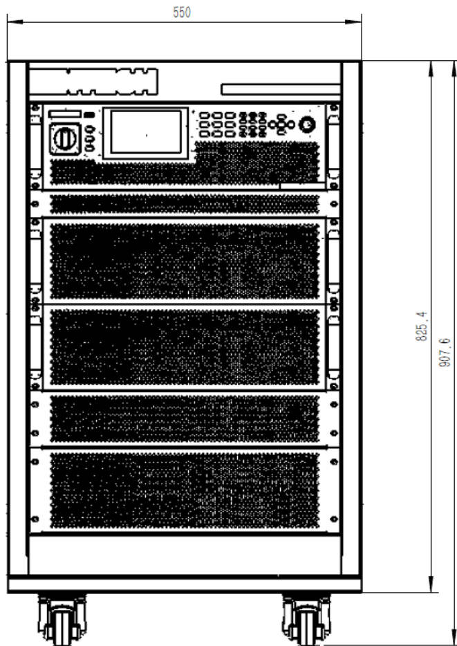
IT7963EP-350-315 机型
