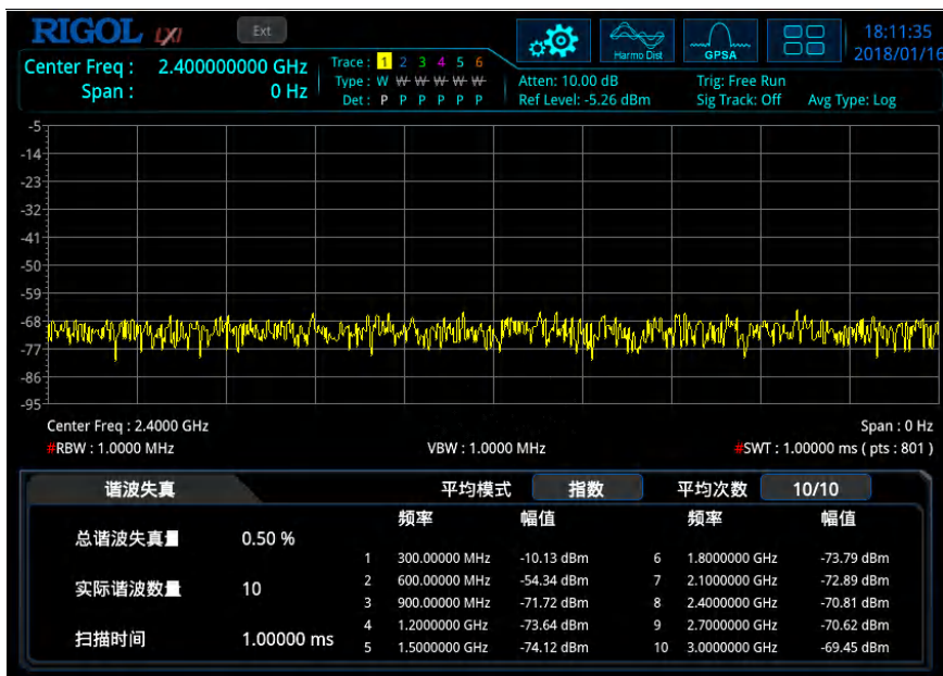
图 2-11 谐波失真测量界面
