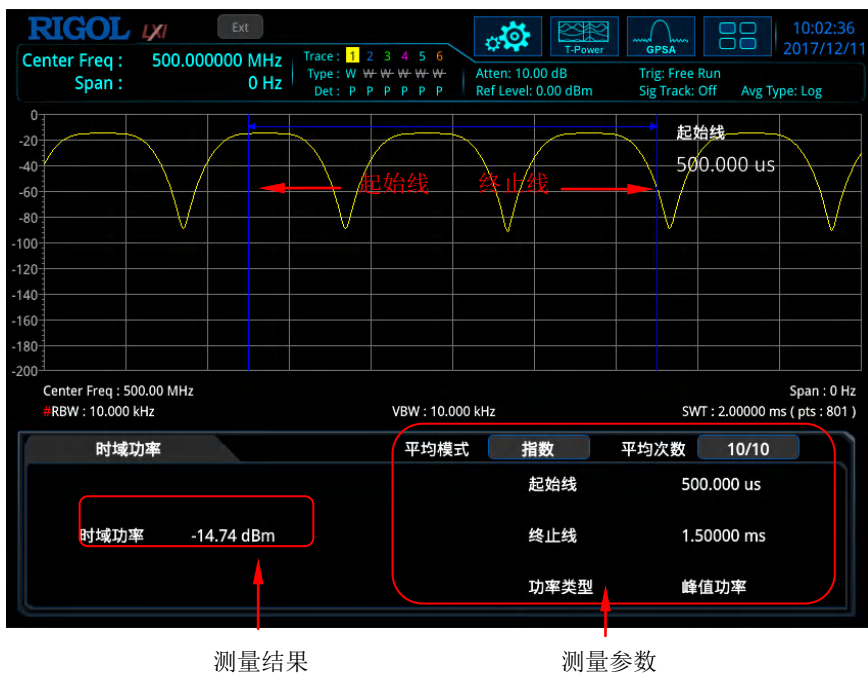
图 2-5 时域功率测量界面
