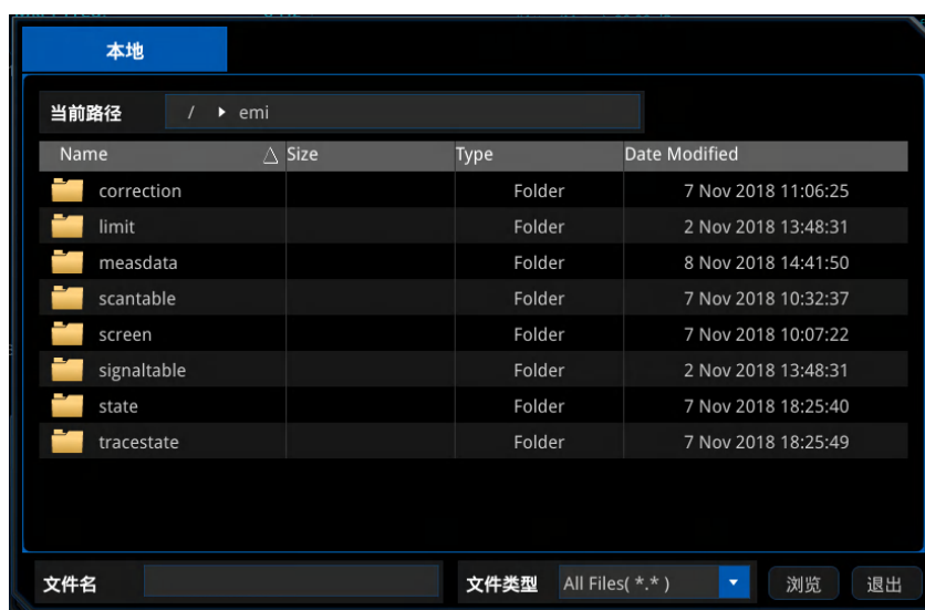
图 4-5 文件管理器
