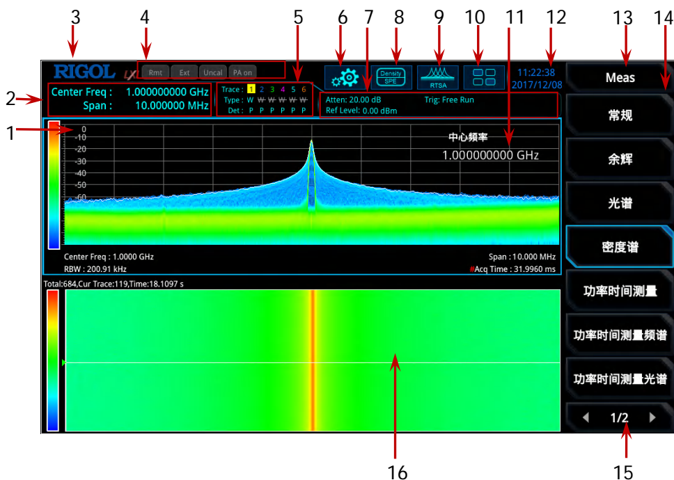
图 1-10 用户界面（RTSA 模式）
