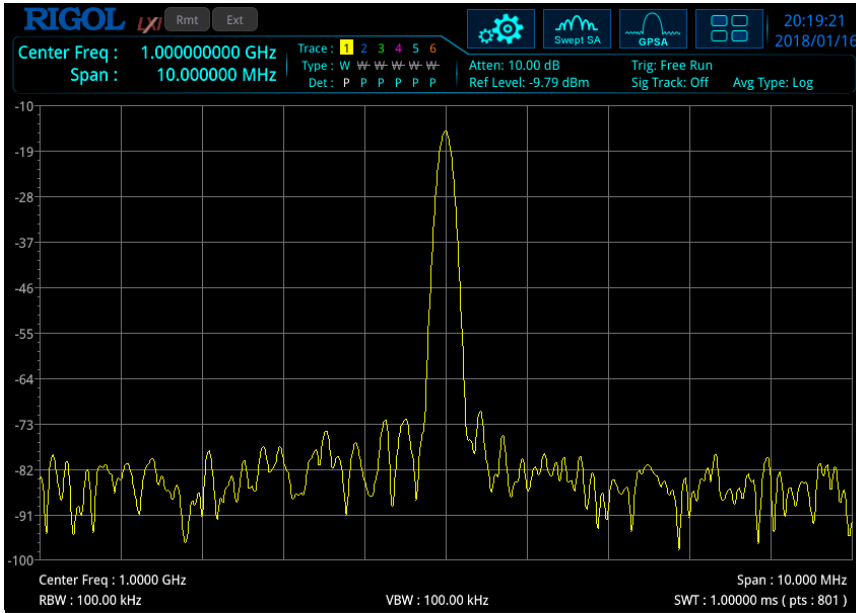
图 2-19 自动搜索信号后
