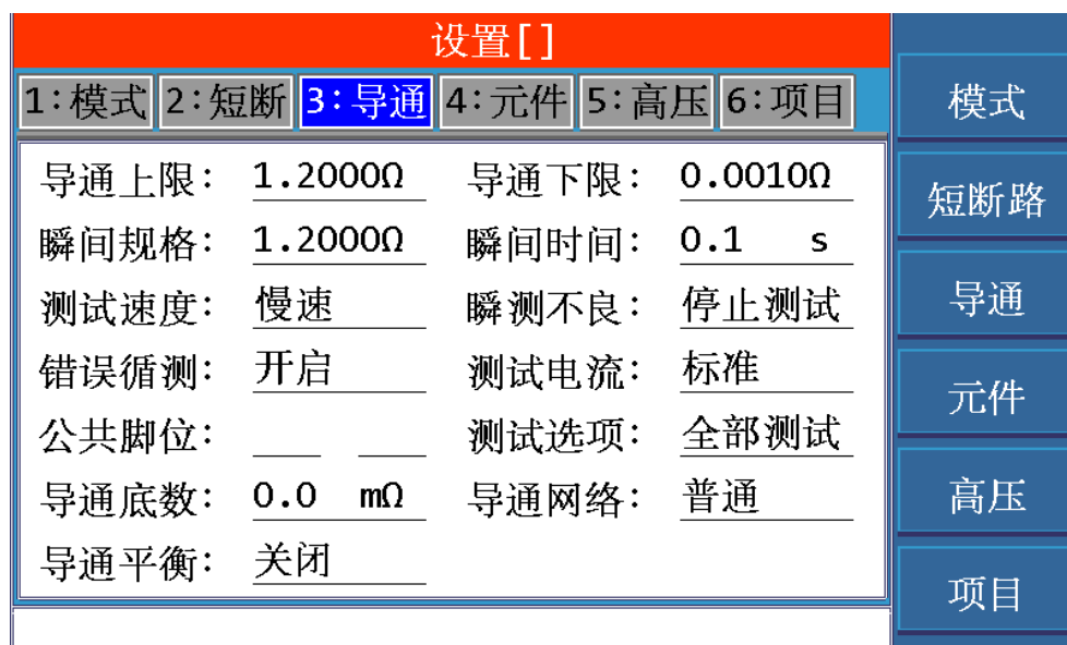
图 3.3-3 导通界面
