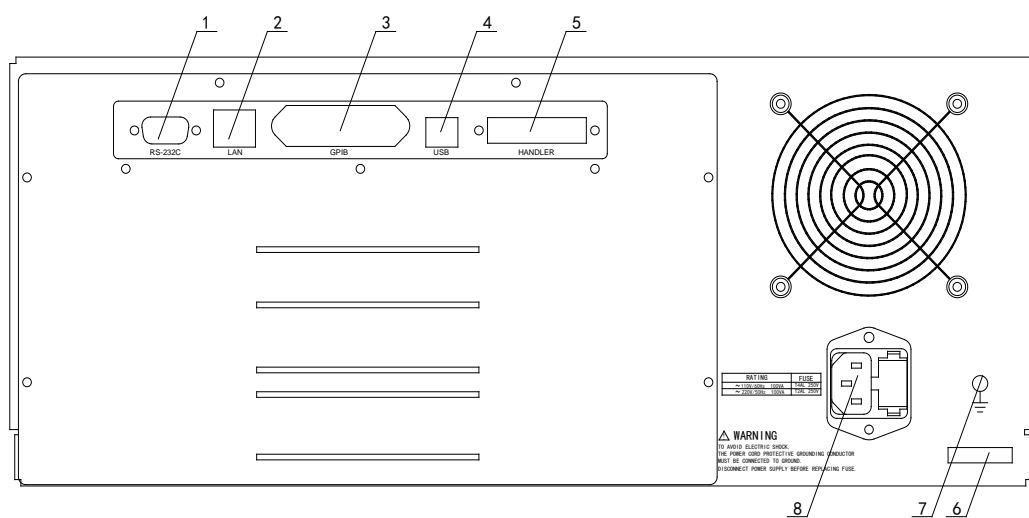
图 2-2. 后面板说明
