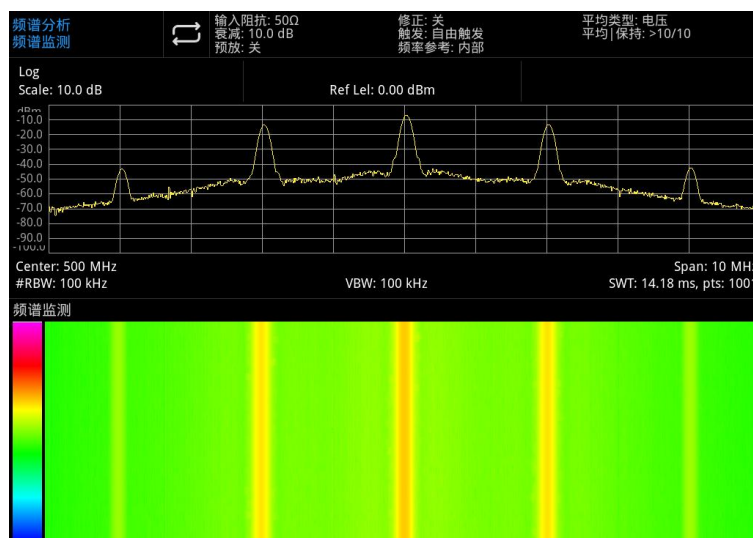
图 5-6：频谱监测
