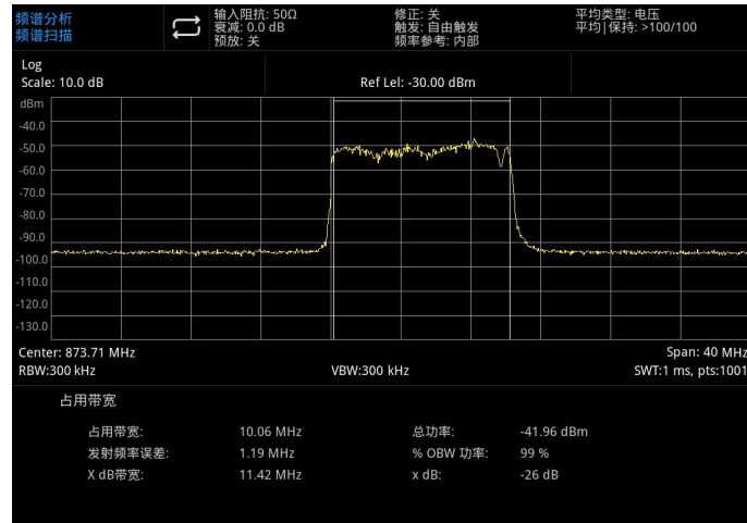
图 5-3:占用带宽
