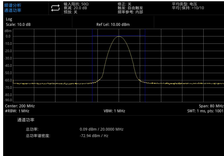
图 5-1: 通道功率
