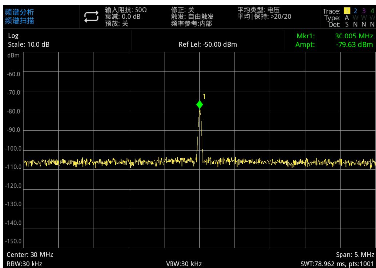
图 3-14: 迹线平均
