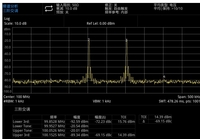
图 5-4：三阶交调
