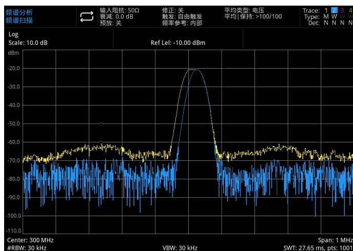
图 3-15：用最大保持和刷新来观察信号飘移
