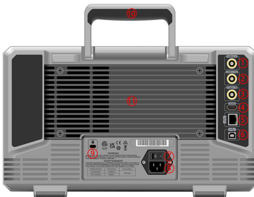
图 1-3: 后面板
