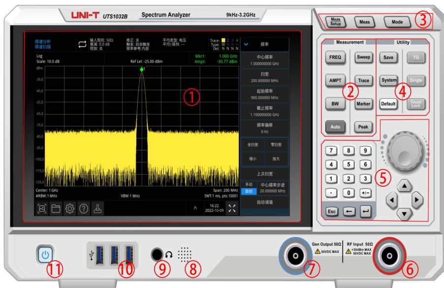
图 1-1: 前面板
