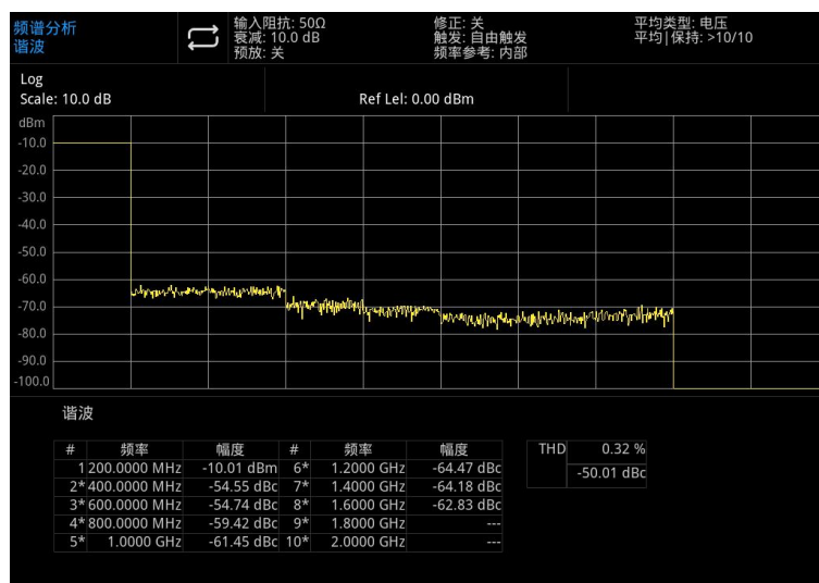
图 5-8：谐波测量
