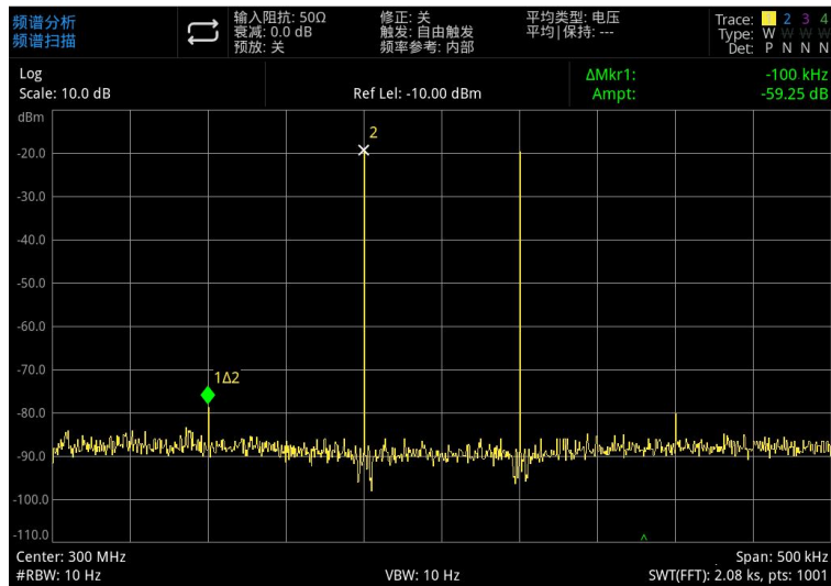
图 3-19: 测量失真产物
