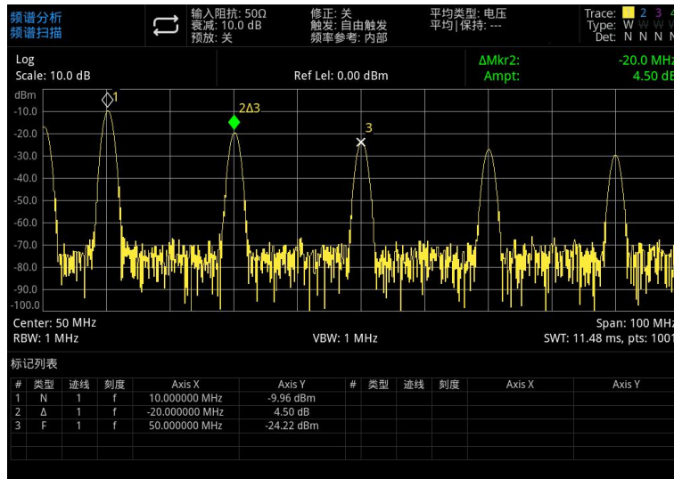
图 4-2: 标记列表
