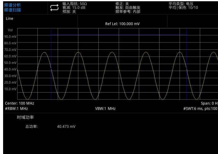
图 5-2：时域功率
