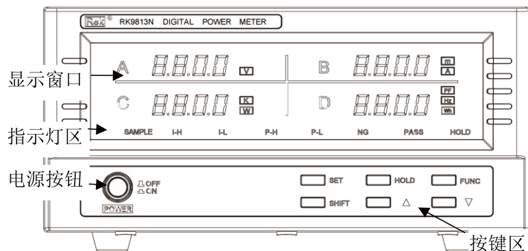
图 1 前面板
