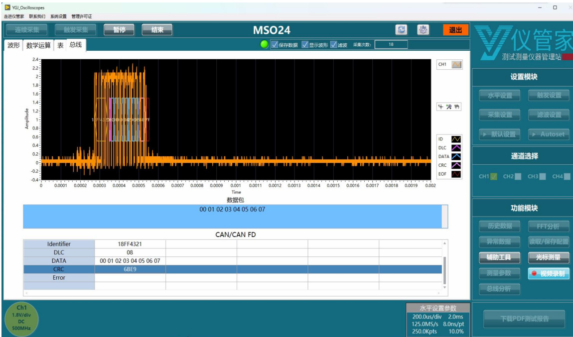
图 5.0-2 功能（二十三）CAN-FD总线解码
