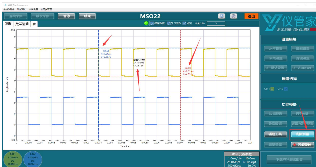
图3.6 功能（二）实时光标测量模式
