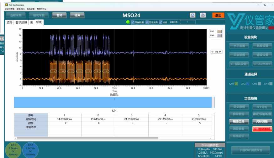
图 4.9 - 3 功能（二十一）SPI总线解码
