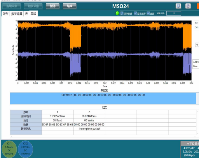
图 4.9 - 2 功能（二十）I2C总线解码
