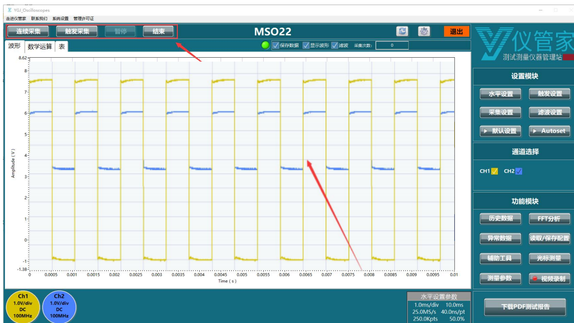
图3.5 功能（一）波形采集和记录
