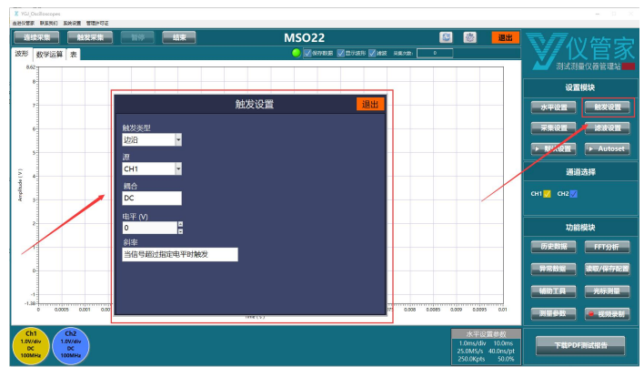
图 4.2 功能（八）设置模块
