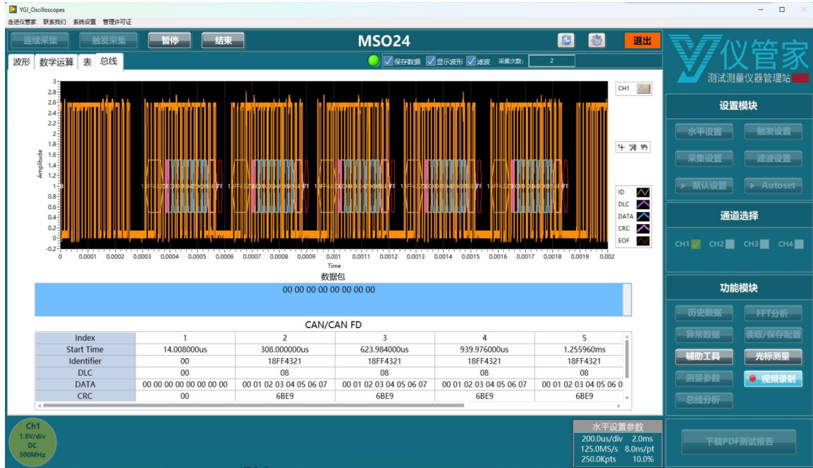
图 5.0-1 功能（二十二）CAN总线解码
