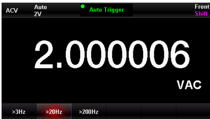
图 2-6 设置低频滤波
