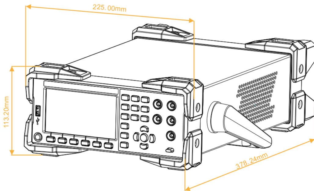
图 1 - 4 外观尺寸
