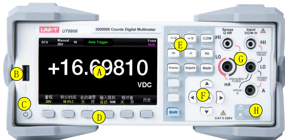
图 1-5 前面板示意图
