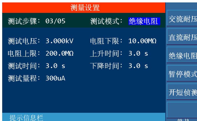
图 4-14 绝缘电阻设置
