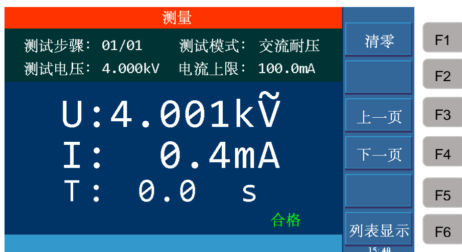
图 4-19 步骤显示界面
