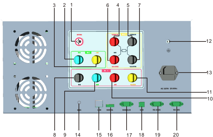
图3-2 RK9970后面板
