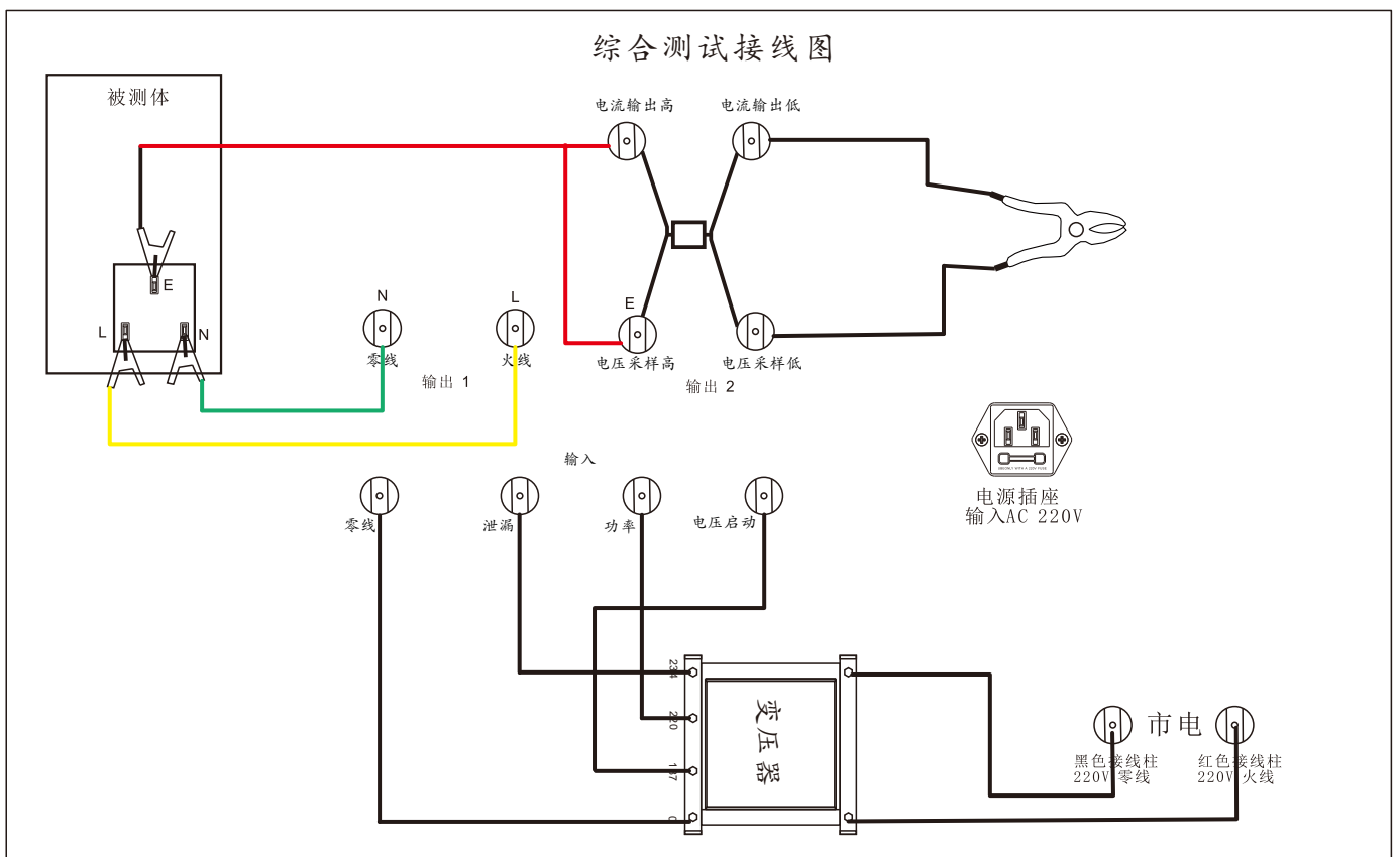
外部接线图
