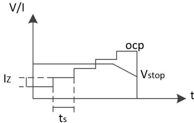
图 5-24 过流测试
