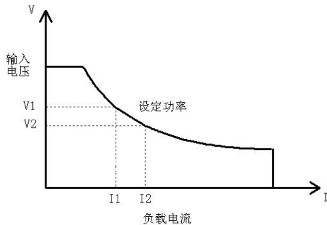
图 5-10 恒功率模式
