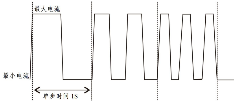
图 5-20 动态扫描
