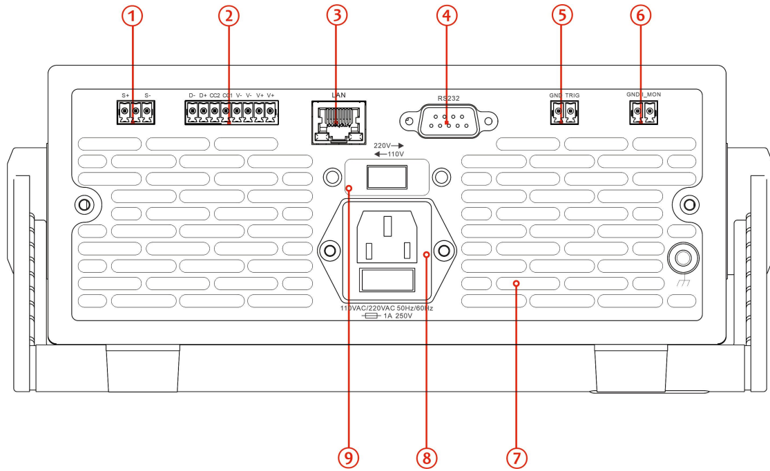
图 4-10 主机后面板
