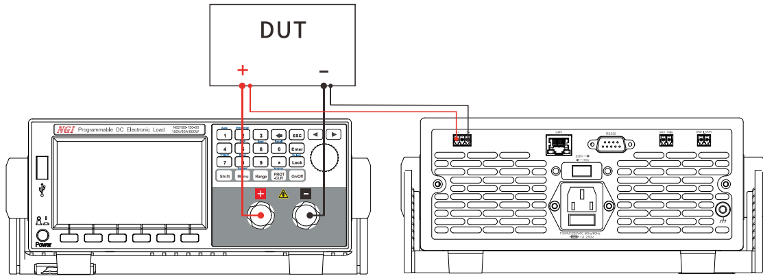
图 3-2 远端采样连接（前后面板接线示意图）
