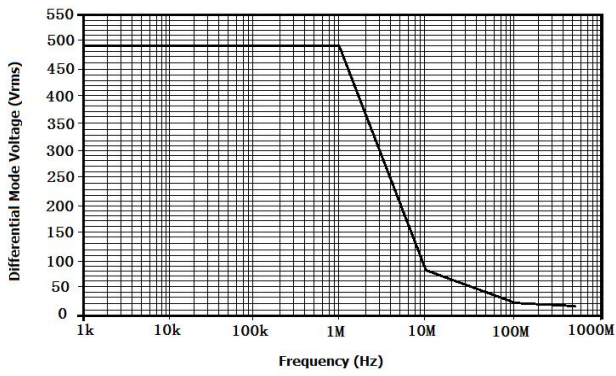
图 1 DP6070B 最大差模电压 VS 频率
