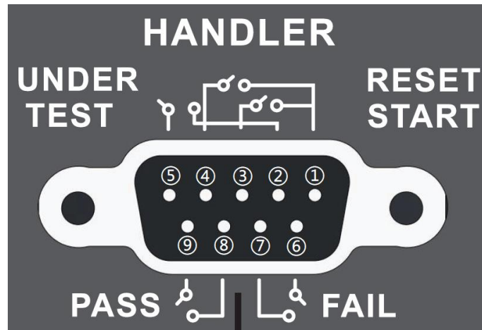
图 8-1 HANDLER 接口图
