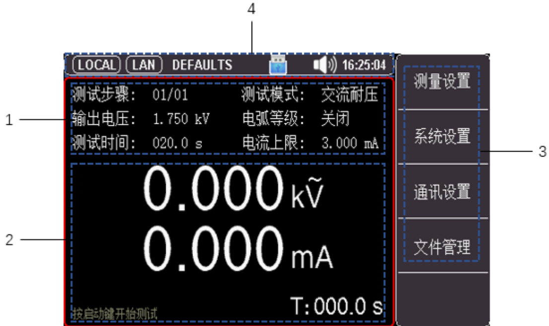
图 4-1 测试显示界面
