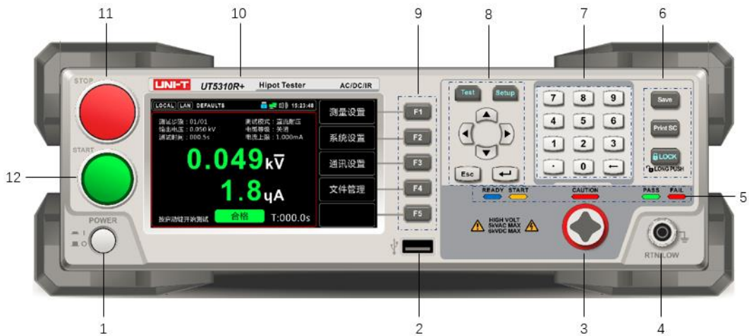
图 1-2-1 前面板介绍 (以 UT5310R+为例) (适用于 UT5310A+/D+/R+/UT5320R+)
