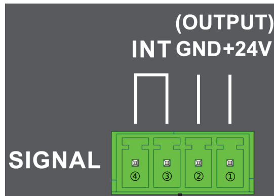
图 8-3 SIGNAL 接口图
