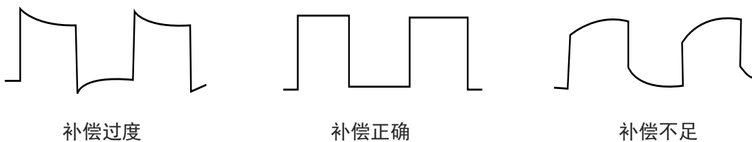
图 4-2 探头补偿校正
