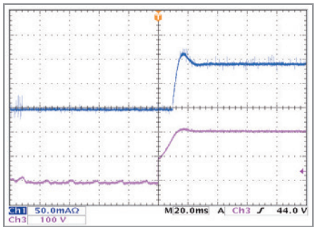
图 6 - LED电源开机波形
