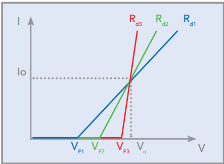
图 3 - 不同特性LED模拟
