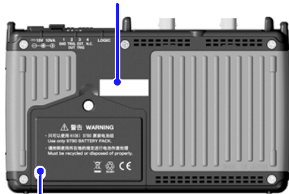
电池组收放盖 (⇒ 第 24 页) 在内部安装选件 9780 电池组。
