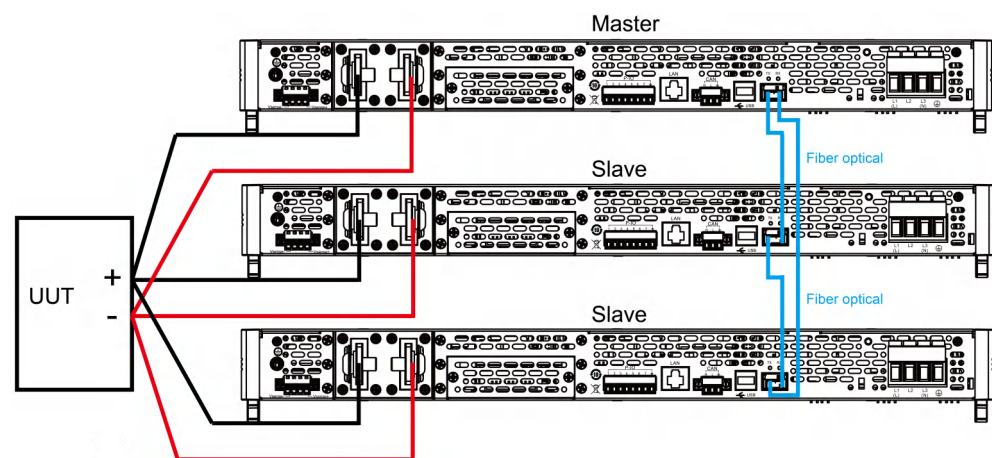
图 5-1 线路连接图
