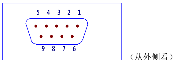
图 5-1 RS232 接口引脚图
