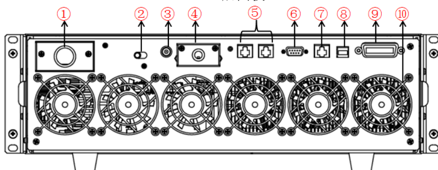
IT7326/IT7326H 后面板
