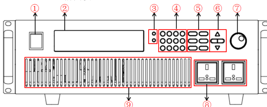
IT7322/IT7324 前面板
