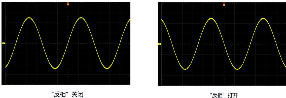
图 5.2 波形反相
