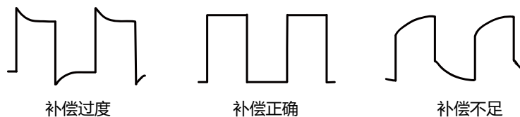
图 4.8 探头补偿
