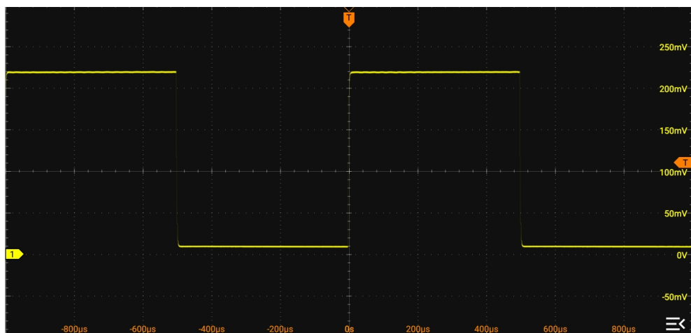
图 4.7 方波信号
