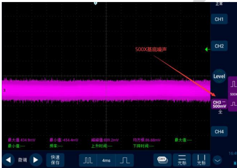
典型值=889mV@500X、4ms/格
