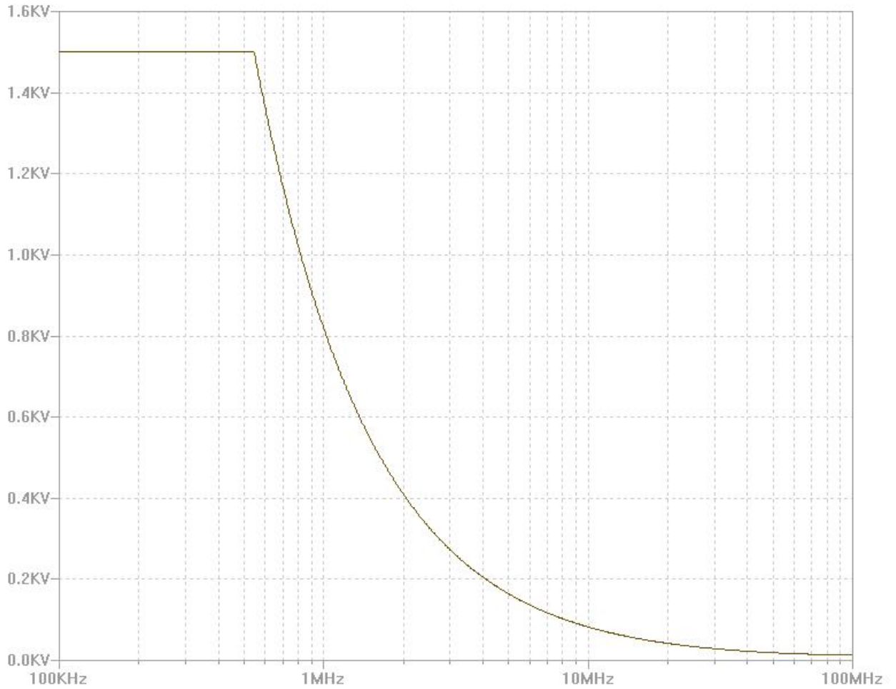
典型差分输入端频率和电压关系图
