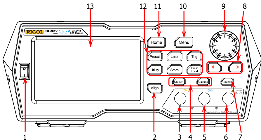
图 1-1 前面板
