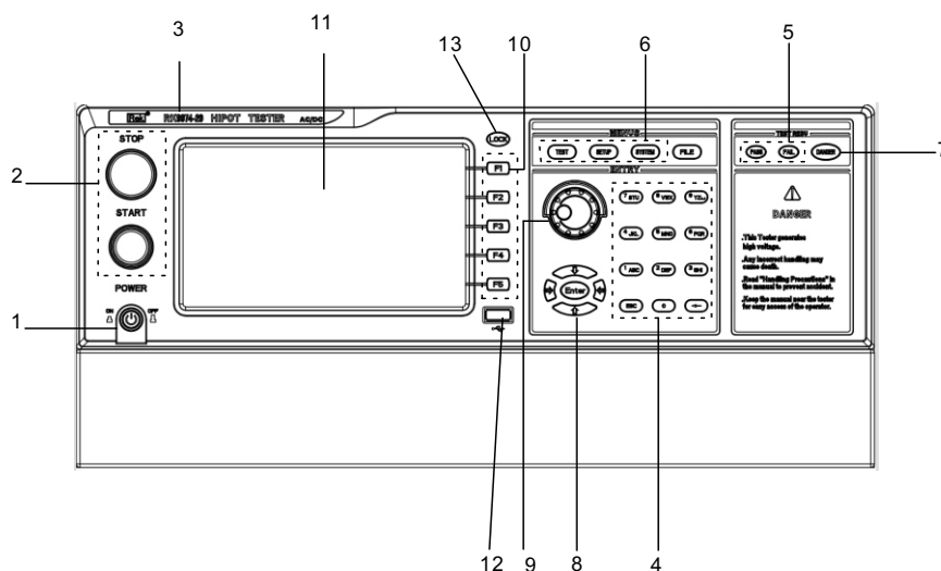
图 3-3前面板说明
