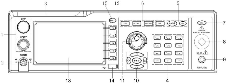
图 3-1 前面板说明
