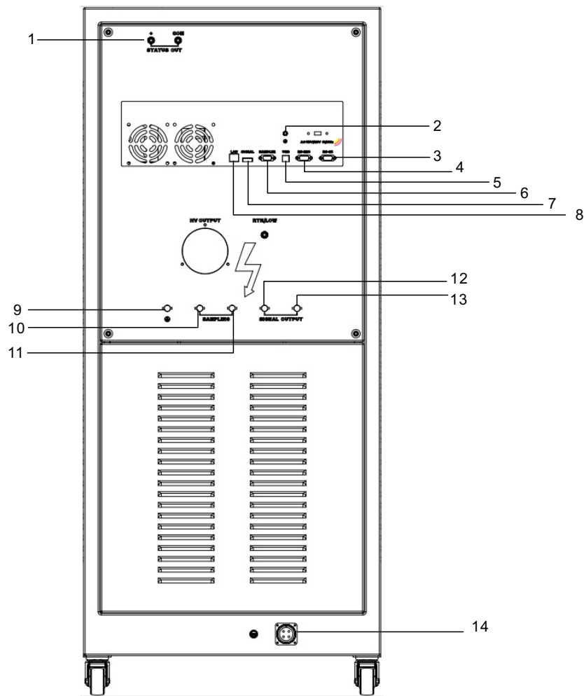
图3.7 后面板说明
