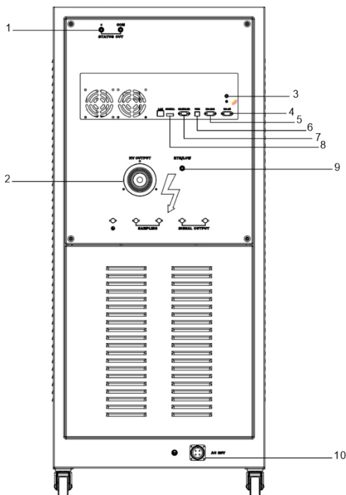
图 3.6 后面板说明
