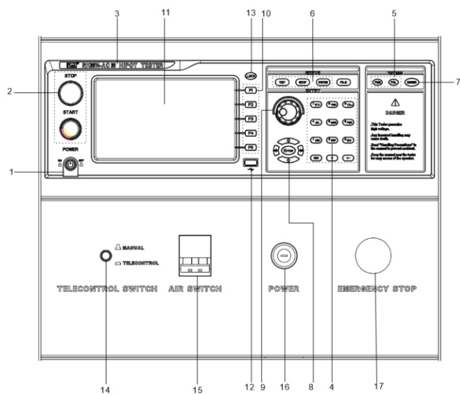
图3.5 前面板说明
