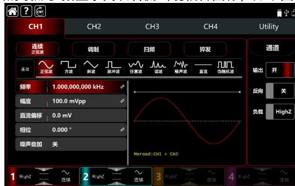
图 2-15 通道耦合
