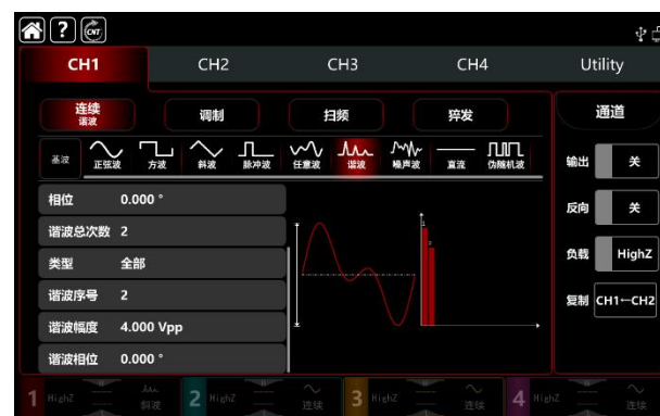
图 2-12 谐波设置
