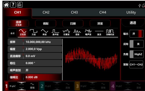
图 2-14 噪声叠加
