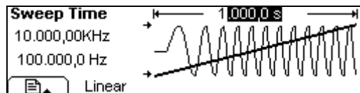
图 3-11 输出线性扫描波形
