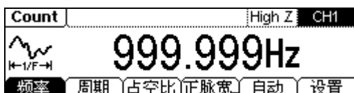
图 2-62 频率计设置界面
