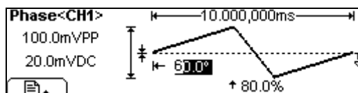
图 3-3 输出锯齿波形
