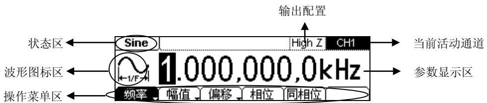
图 1-5 单通道常规显示模式
