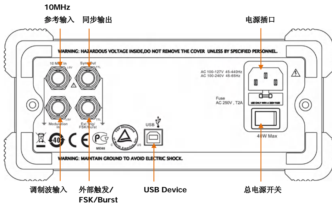
图 1-4 后面板
