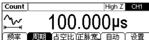
图 3-26 周期测量值
