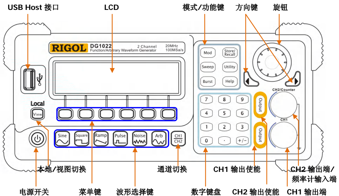
图 1-3 前面板
