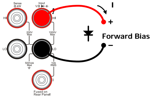
图 2-29 二极管检测示意图
