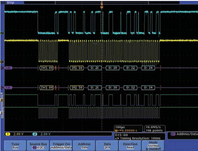
图55. 自动触发、解码和搜索串行数据包上下文加快了串行总线分析速度。
