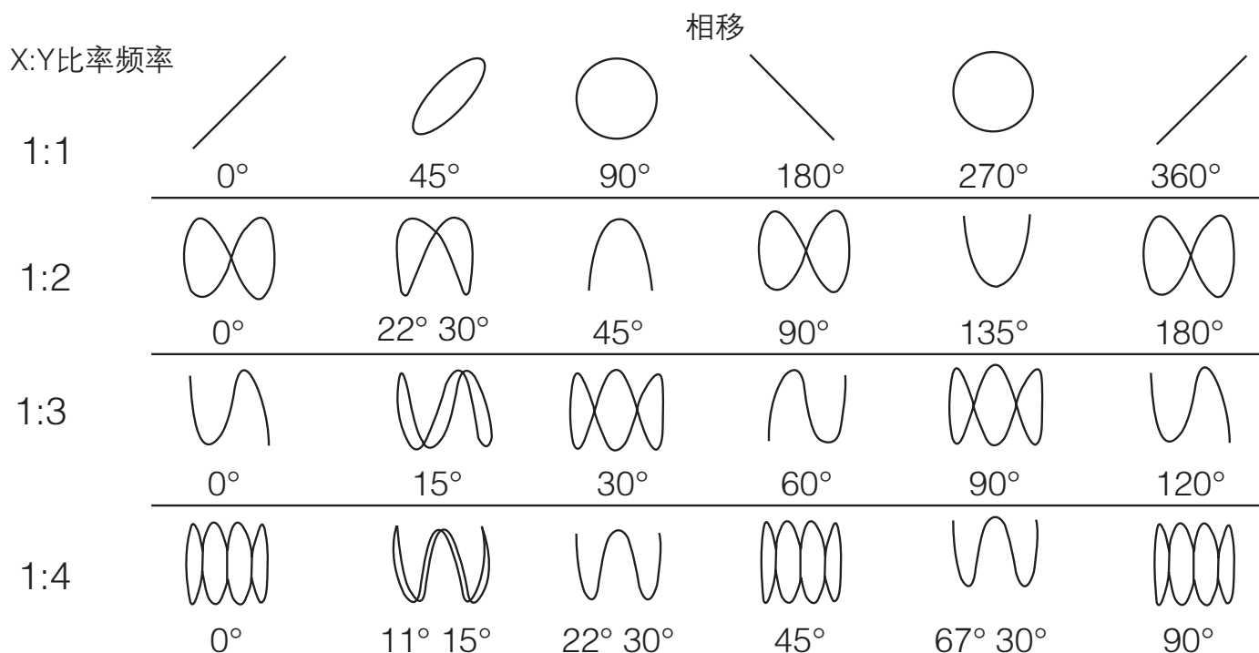
图70. Lissajous码型。
