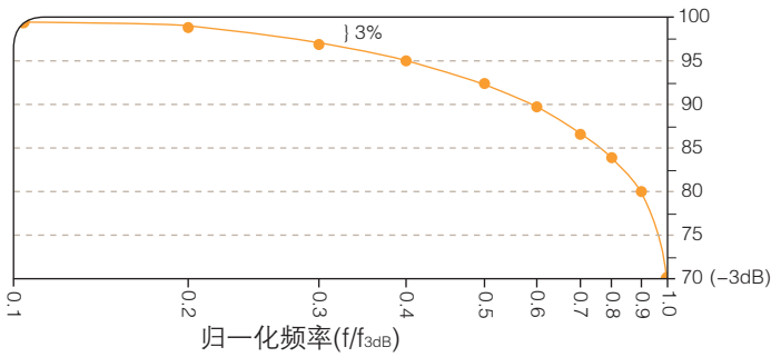
图44. 示波器带宽是正弦曲线输入信号被衰减到信号实际幅度70.7%的频率，称为-3 dB点。
